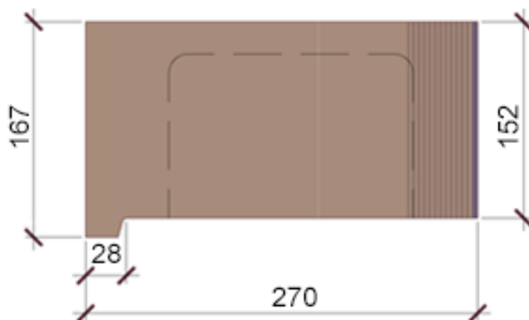
Рисунок 2.2. Подпорный камень. Вид сбоку.
