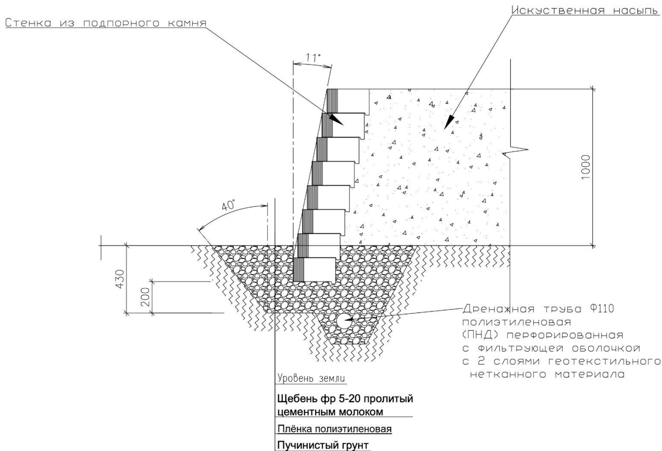
Рис.3.1.1. Подготовка площадки в условиях гладкого рельефа
