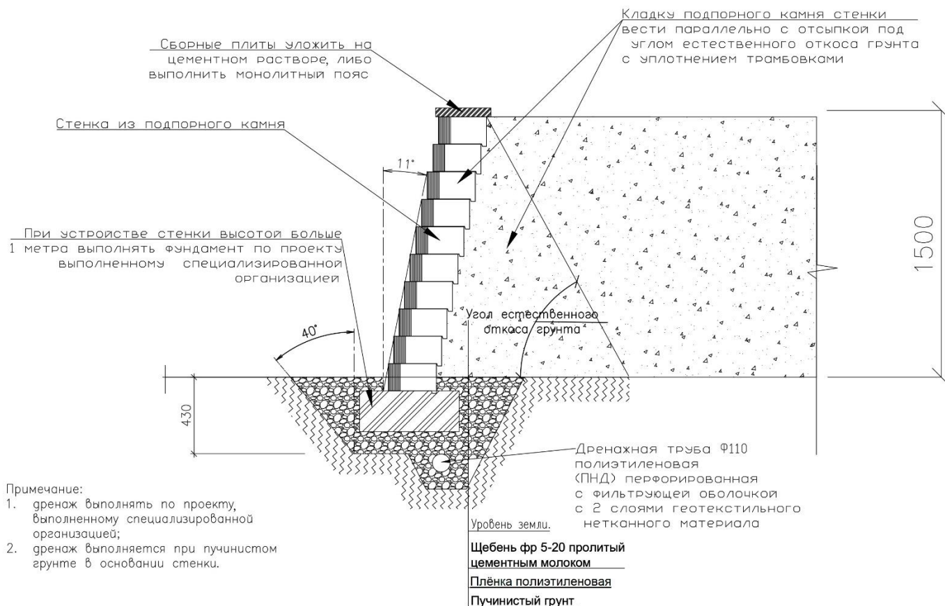
Рис. 3.5 Устройство подпорной стенки высотой 1-1,5м
