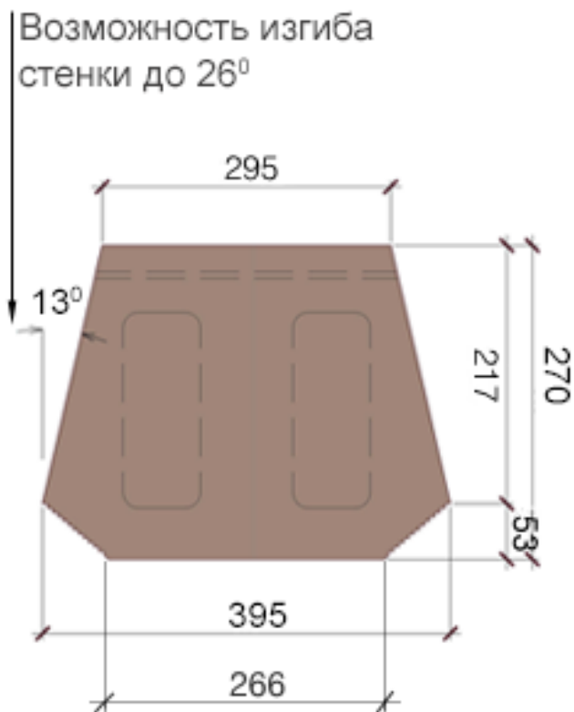
Рисунок 2.3. Подпорный камень. Вид сверху (монтажное положение)
