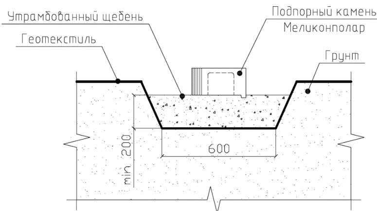
Рис. 3.4. Устройство основания для подпорной стенки высотой до 1 м (непучинистый грунт)
