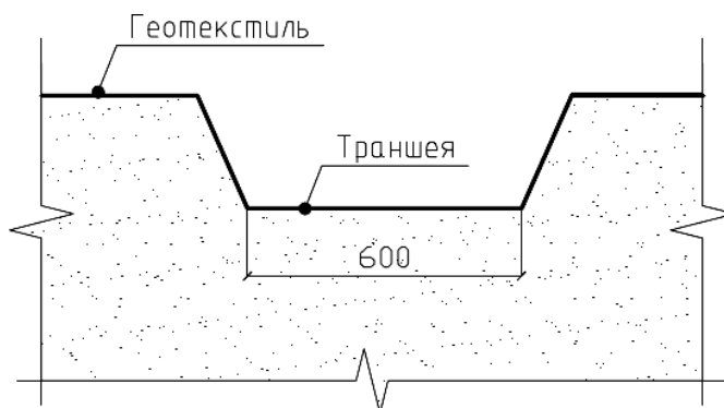
Рис.3.2. Траншея
