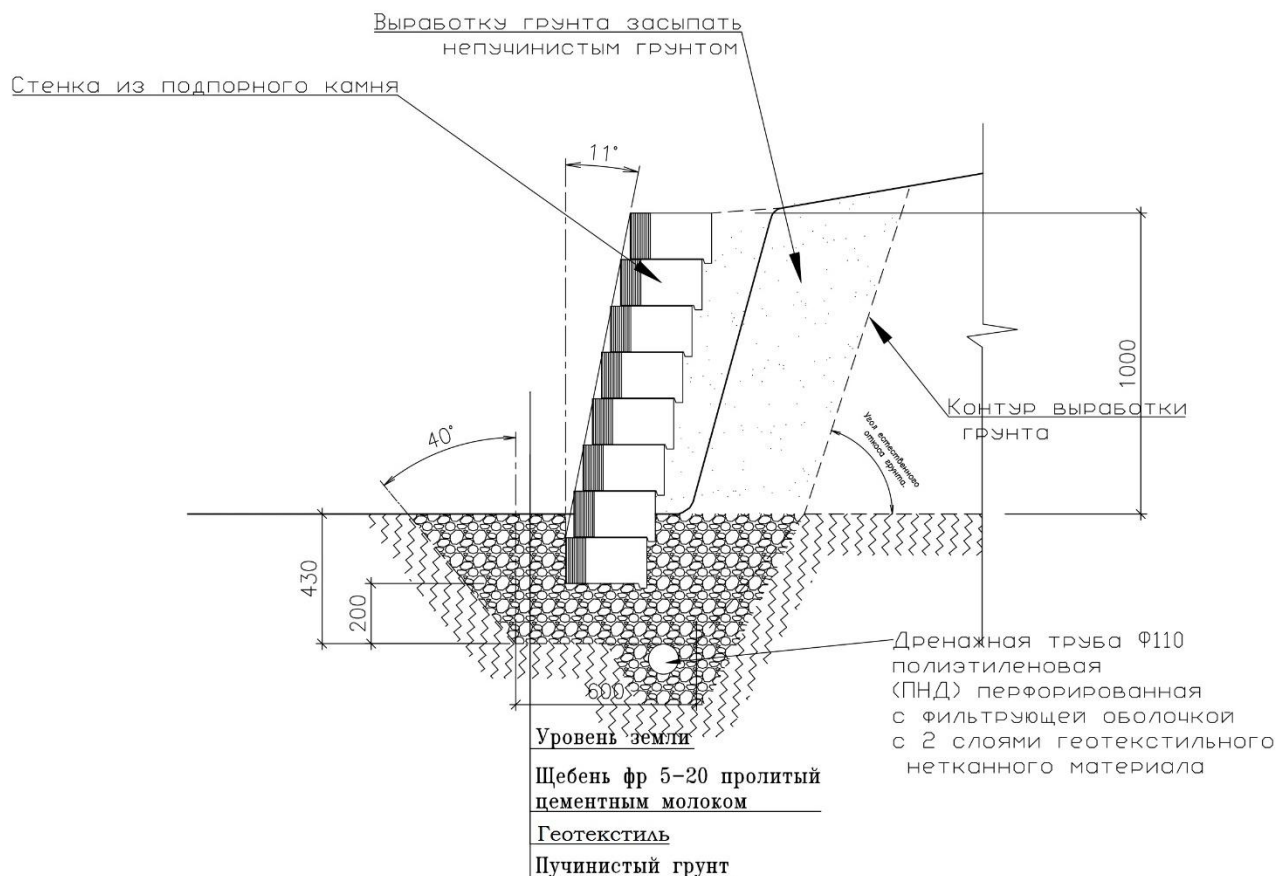
Рис.3.1.2. Подготовка площадки при условии значительного перепада высот
