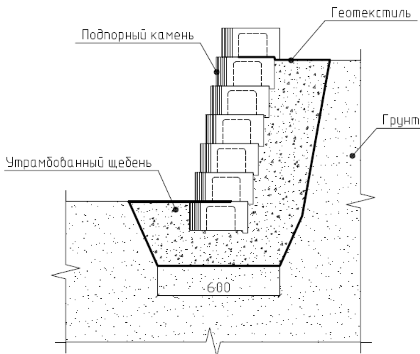
Рис. 3.3. Схема укладки геотекстиля
